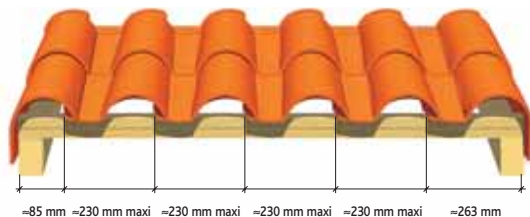
Pose avec tuile de rives à rabat
