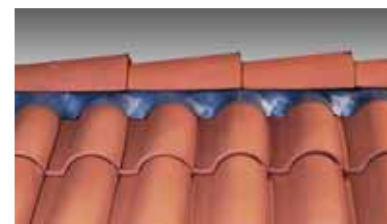
Faitage réalisé à sec avec faîtière à pureau variable et closoir ventilé, sans emploi de mortier.
