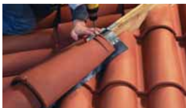
Après coupe des tuiles d'approche, pose du closoir ventilé sur lisse de rehausse et fixation des arêtiers par clips.
