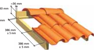
Faîtière pureau variable et tuile sous-faîtière pureau entier.
