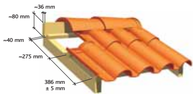
Faîtière pureau variable et tuile sous-faîtière 2/3 pureau.
