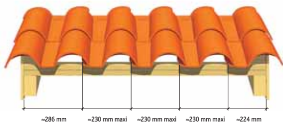
Pose sans tuile de rives à rabat
